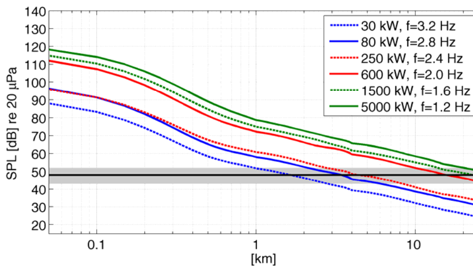
Abbildung 7: Verlauf des emittierten Schalldruckpegels (SPL) mit der Entfernung zur Quelle für die 2. Flügelharmonische. Die baulichen Parameter der Windräder sind Tabelle 1 zu entnehmen. Der grau unterlegte Bereich markiert das Hintergrundrauschen zwischen 1 und 3 Hz an der Infraschallstation I26DE im Bayerischen Wald.
